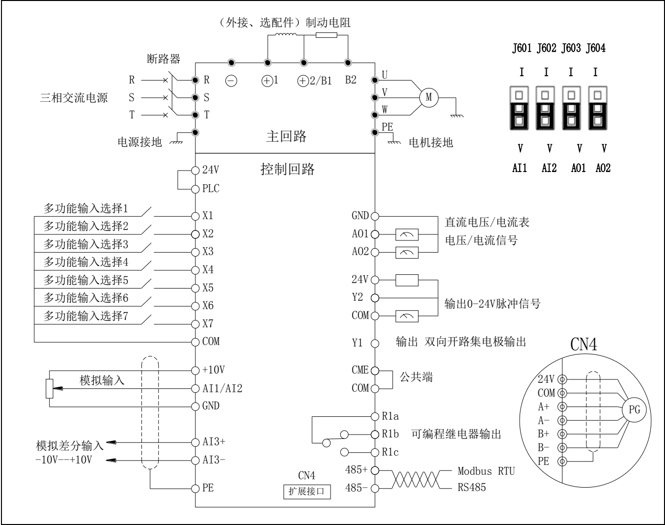
图 4-1 基本配线图
