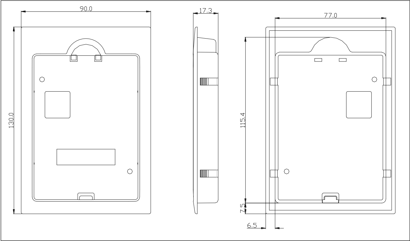
图 2-3 安装盒尺寸
