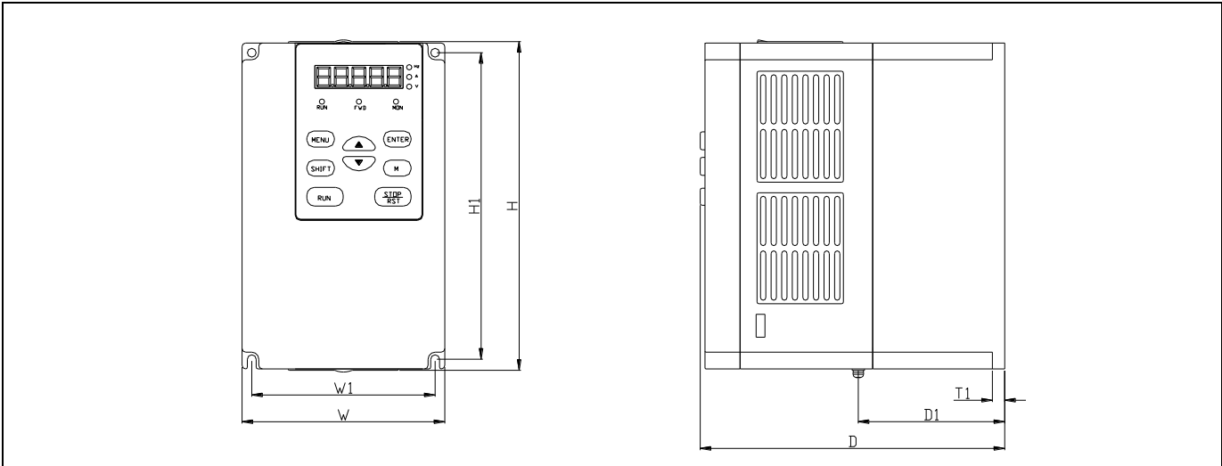
图 2-1 FV100-4T-0037G/0055L 以下功率变频器
