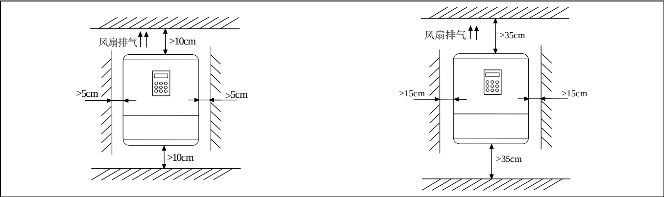
图 3-1 安装的间隔距离(0450G/0550L 及以下) 图 3-2 安装的间隔距离(0550G/0750L 及以上)
